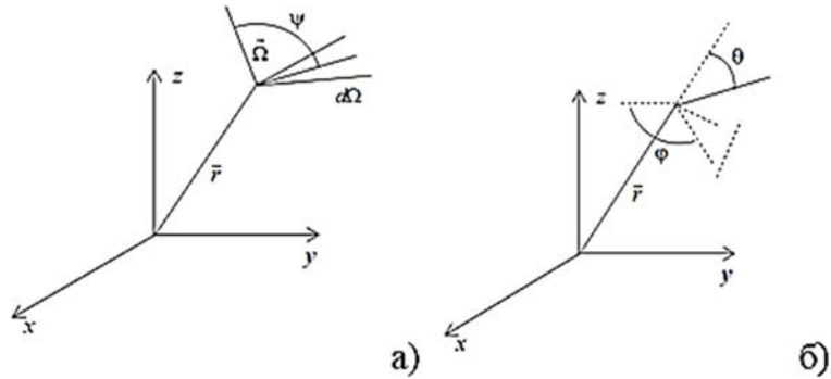
Рис. 2. Основные характеристики направления движения частиц: при рассеянии направления движения частицы меняется с \vec{\Omega} на \vec{\Omega}' (а); выражение декартовых компонент \vec{\Omega} через сферические координаты (б) [5]
