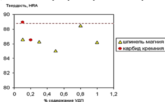
Рис. 1. Зависимость твердости по Роквеллу опытных образцов буровых пластин от содержания ультрадисперсных модификаторов
