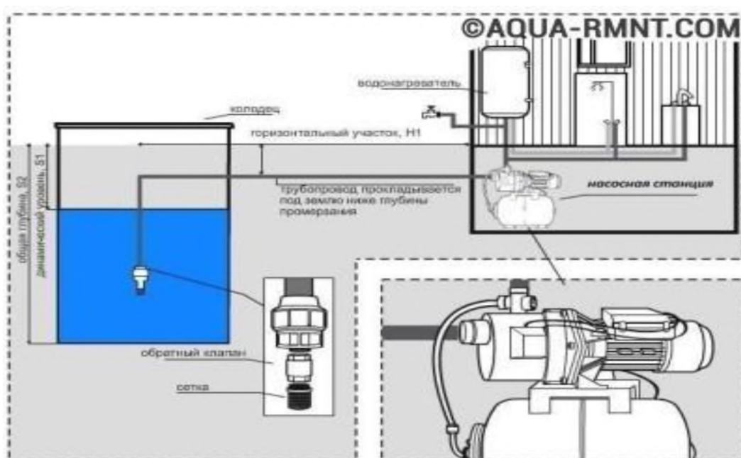
Рисунок 1 - Схема установки насосной станции в частном доме
