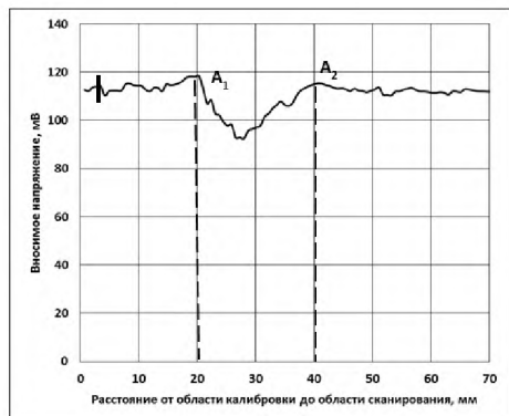
Рис. 2. Результаты измерений для сварного шва с дефектами, область 1.
