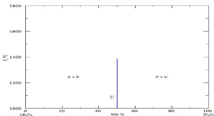
Рисунок 1 – Диаграмма состояния \text{La}_2\text{O}_3 - \text{In}_2\text{O}_3
