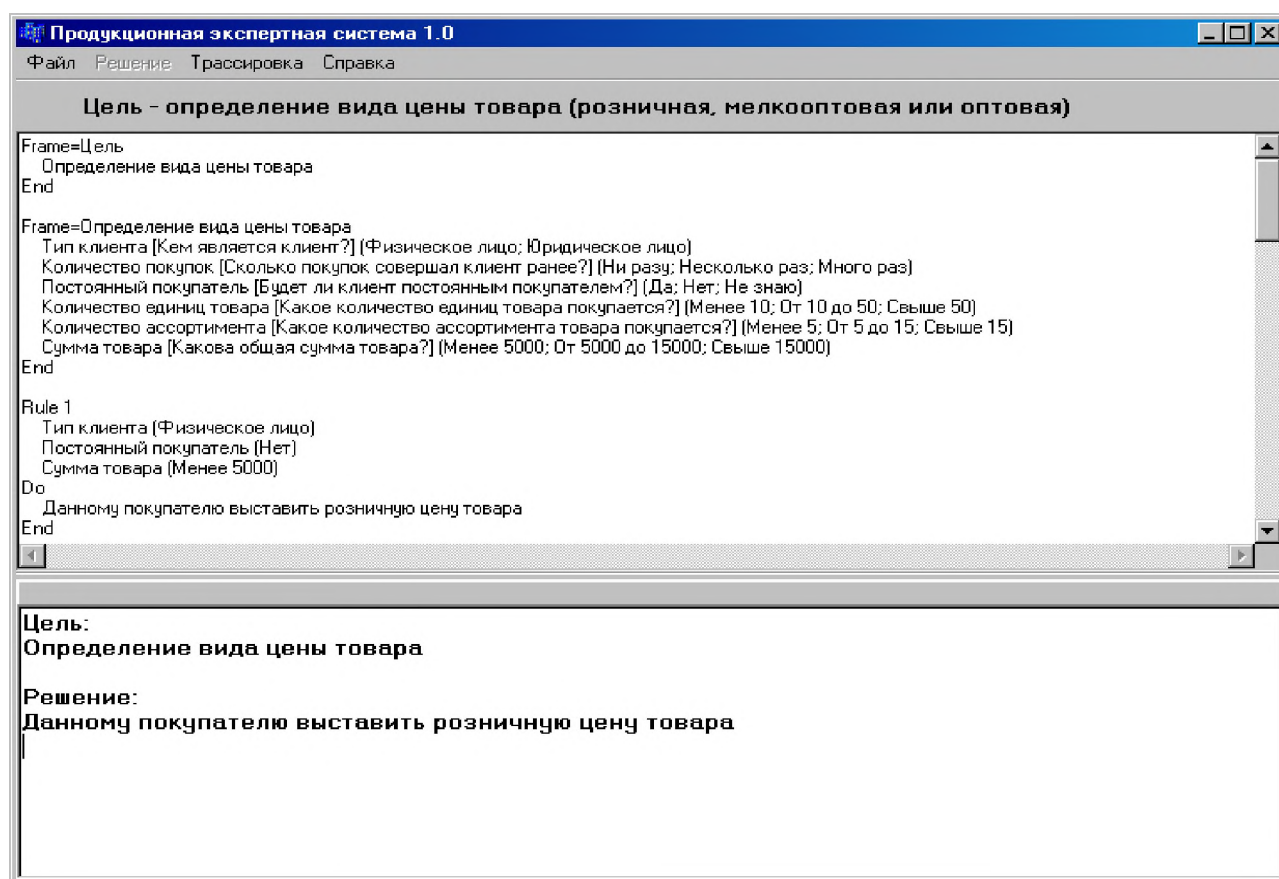
Рисунок 1 – Пример работы продукционно-фреймовой модели экспертной системы
