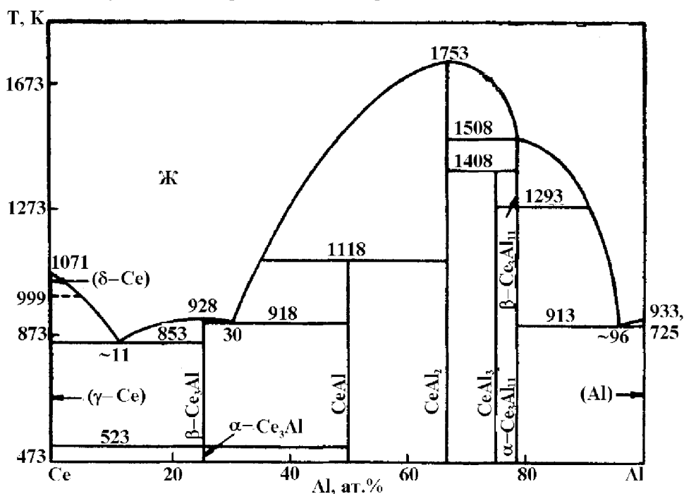
Рисунок 1- Диаграмма состояния Al-Ce
