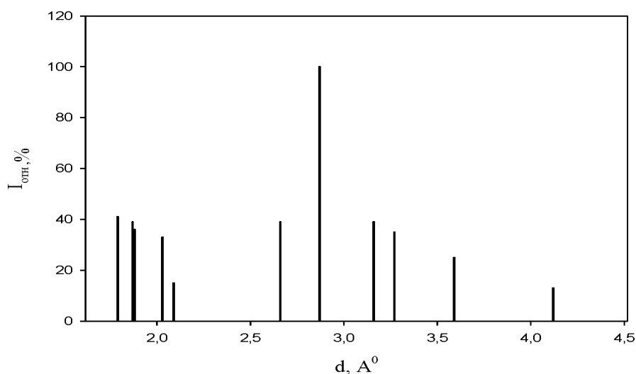
Рисунок 2 – Штрихрентгенограмма \text{LaInO}_3 (экспериментальные данные)
