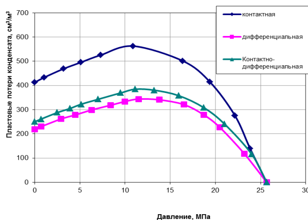
Рис. 1. Кривые пластовых потерь углеводородов при изотермической конденсации газоконденсатной системы.
