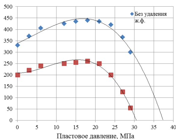
Рис. 2. Аналитические прогнозные кривые пластовых потерь конденсата залежи БУ 8 1-2
