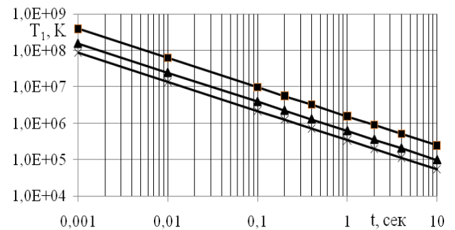
Рис. 1. Зависимости температуры T_1 от времени t на фронте УВ в фотосфере при E = 4,19 \cdot 10^{24} Дж, \tau = 180 сек и разной начальной плотности \rho_0 = 10^{-4}, 10^{-5}, 10^{-6} кг/м 3 - звезды, треугольники, квадраты.
