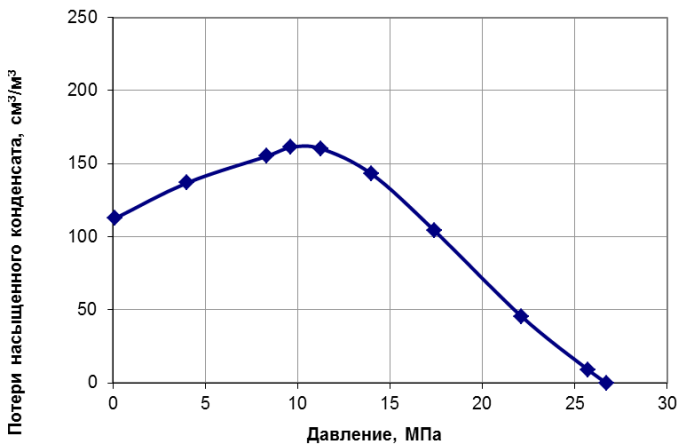
Рис. 2. Кривая зависимости пластовых потерь конденсата от давления, полученная методом дифференциальной конденсации.
