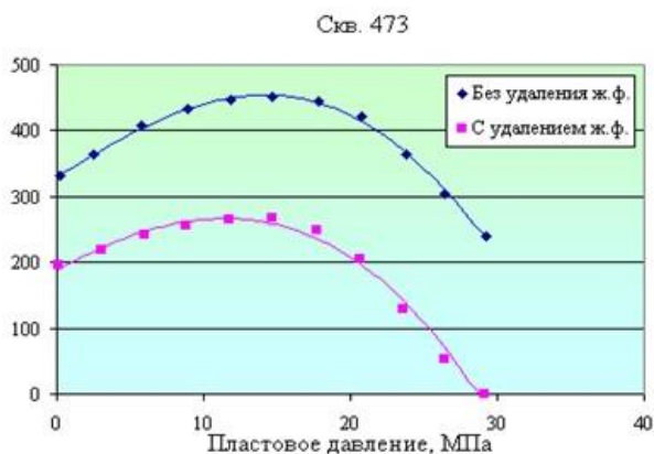
Рис. 1. Экспериментальные кривые пластовых потерь газоконденсатных смесей пласта БУ 8 1-2
