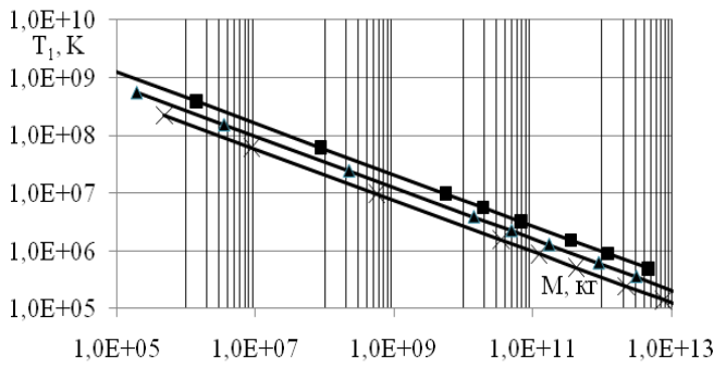
Рис. 2. Зависимость температуры T_1 на фронте от массы M водорода за фронте УВ при взрывах с энергией E_1 = 4,19 \cdot 10^{22} Дж за время \tau = 4,19 сек при разных плотностях \rho_0 . Обозначения как на рис. 1.
