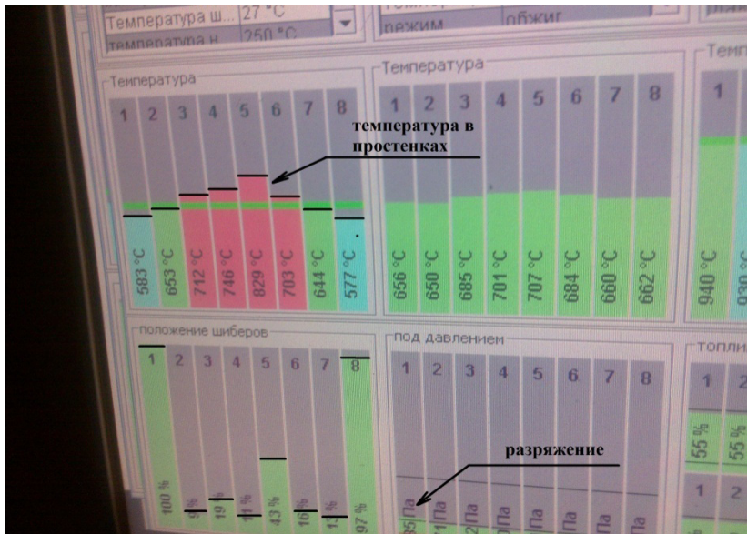
Рисунок 2 — Параметры обжига.
