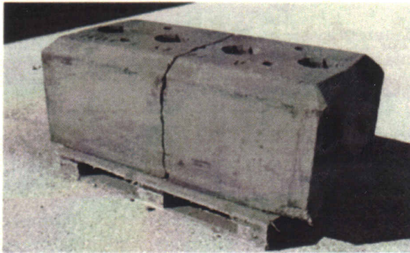
Рисунок 5 — Вертикальная трещина в теле анода.
