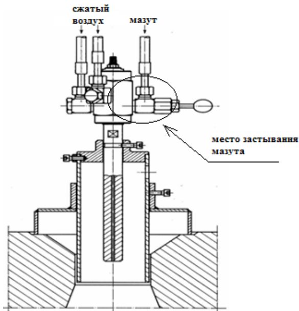
Рисунок 7 — Топливная горелка (указано место закупоривания застывшего топлива).
