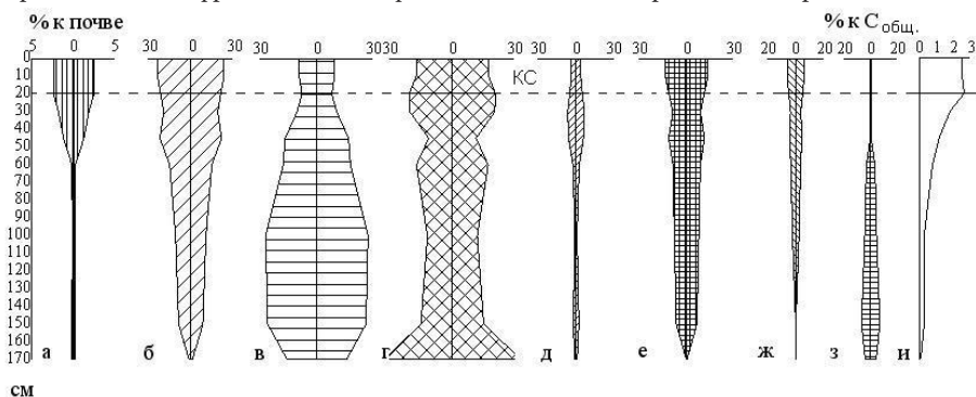
Рис. 1 — Гумусовый профиль погребенных городских почв Екатеринбурга Обозначения: а — общий углерод, % к почве.; % к С общему; б — гуминовые кислоты (ГК), в — фульвокислоты (ФК), г — негидролизуемый остаток (гумин); д — ГК-1; е — ГК-2; ж — ГК-3; з — ФК-1 а; и — Сгк: Сфк
