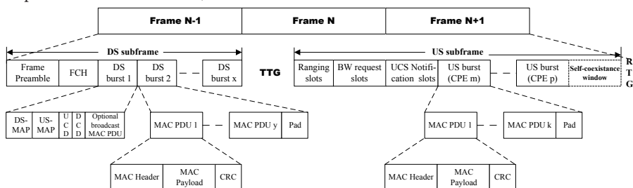
Рис. 3. Структура фрейма
