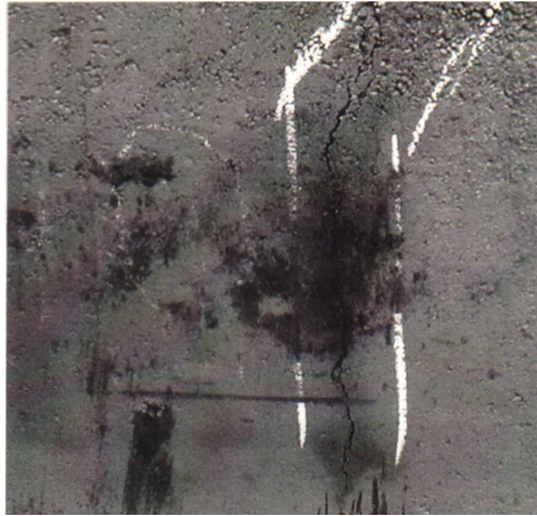
Рисунок 4 — Трещина, образовавшаяся в результате повышенной скорости нагрева.
