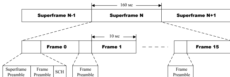
Рис. 2. Структура суперфрейма
