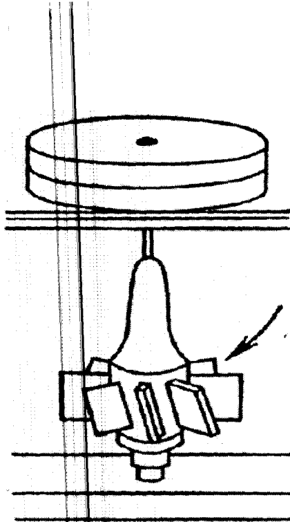
Рисунок 1 - Схема простого водяного колеса с вертикальным валом.
