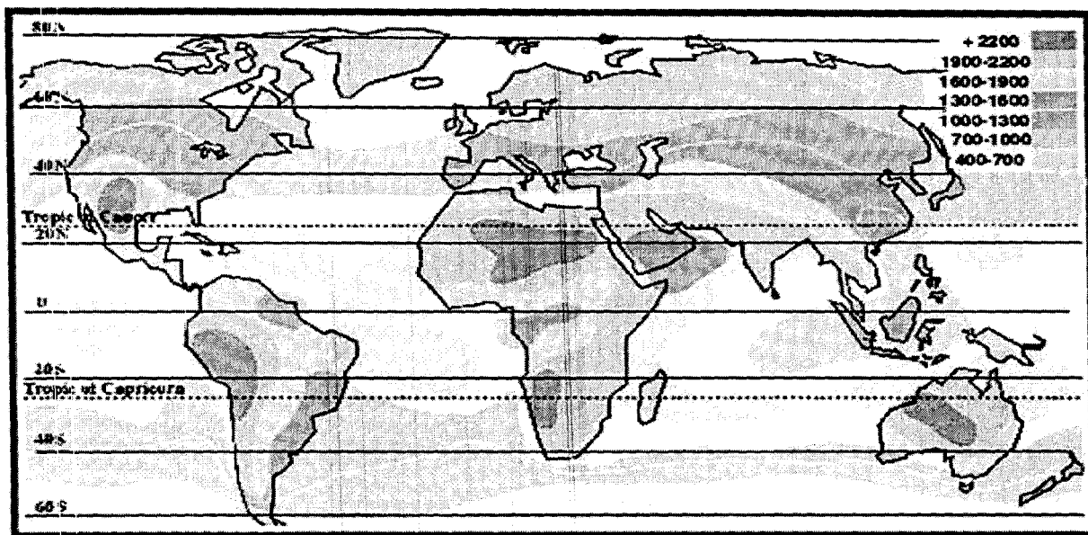
Рисунок 6 - Распределение солнечной радиации на поверхности Земли (кВтч/м 2 /Год)
