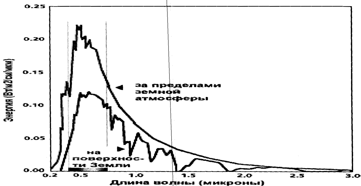
Рисунок 4 - Радиационные волны
